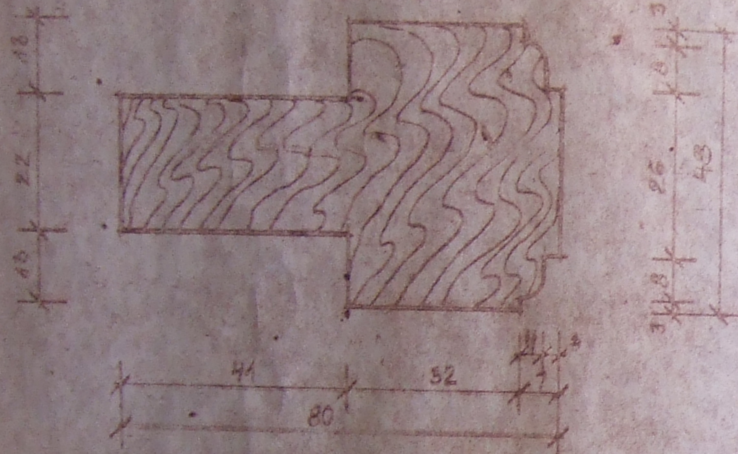
AKNA A-2 IMPOST M 1:1
