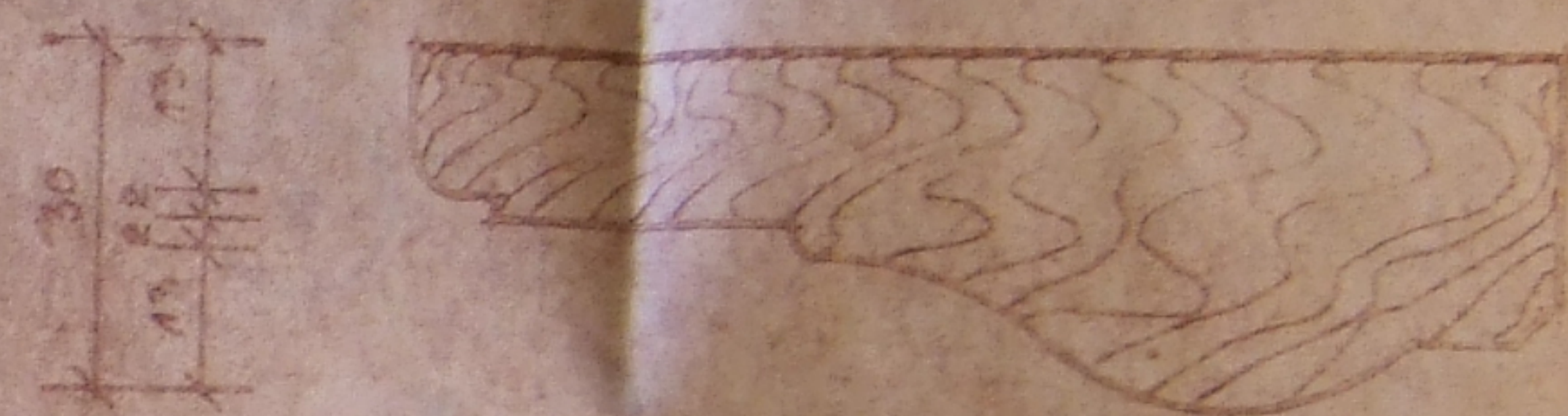
I KORRUSE UKSE PIIRDELIIST M 1:1
